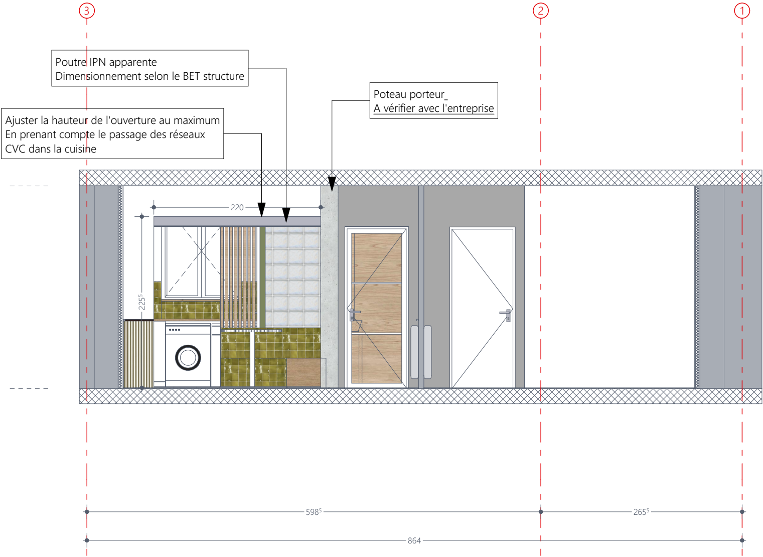
DD' Coupe DD Structure Ouverture 1:50
