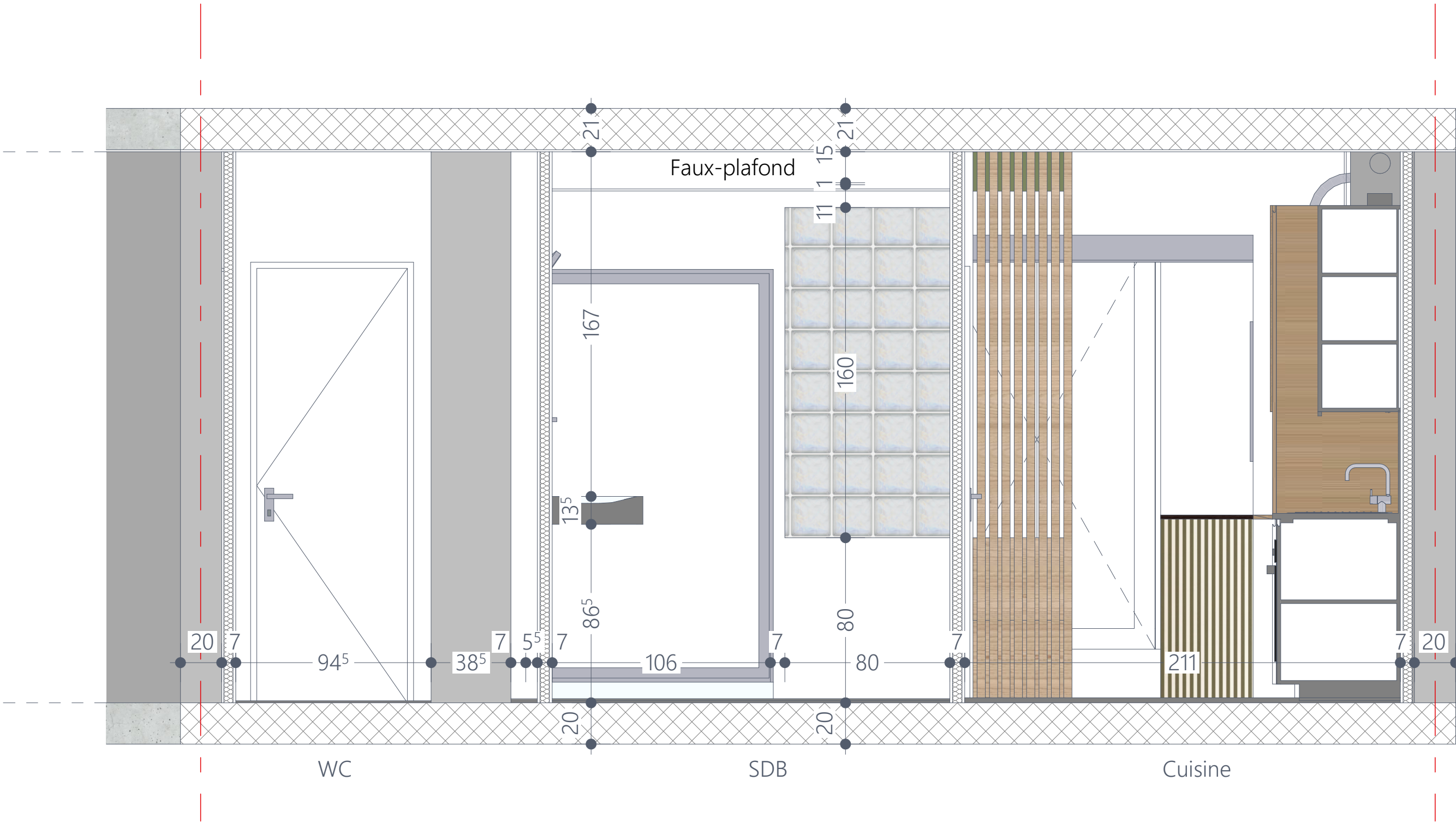
CC' Coupe CC
